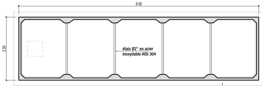
SCHÉMA
